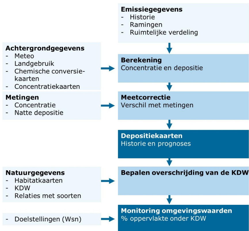
Figuur 4 Schematische weergave van de gehanteerde methode om de stikstofdepositie en de overschrijding van de kritische depositiewaarden te berekenen.
