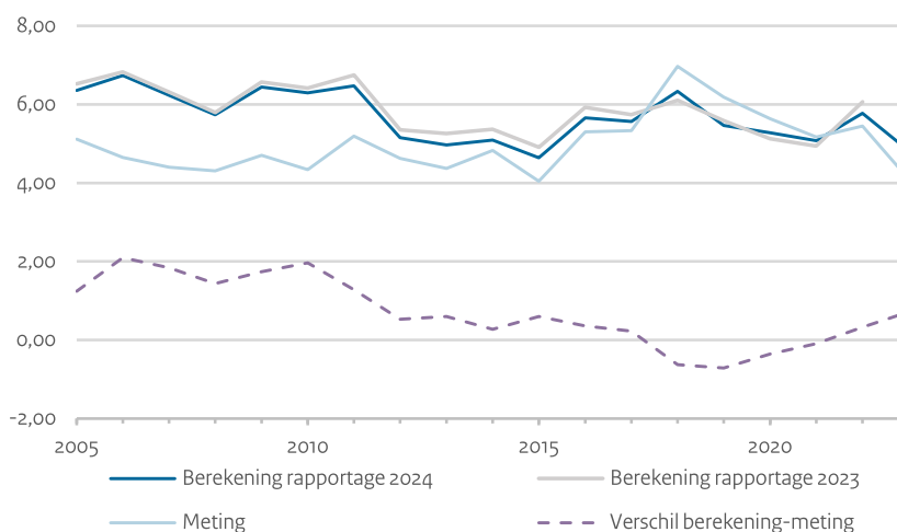
Figuur 35 De gemiddelde berekende en gemeten ammoniakconcentratie 2005-2023 (blauwe lijnen). Het verschil tussen beiden (licht paars) is waar met de kalibratie de berekeningen voor worden gecorrigeerd. De grijze lijn geeft de berekeningen van de vorige rapportage aan.
